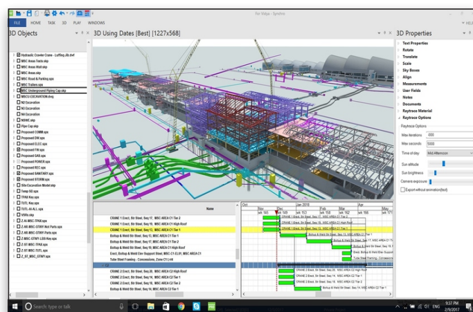
4D-модель проекта аэропорта.
